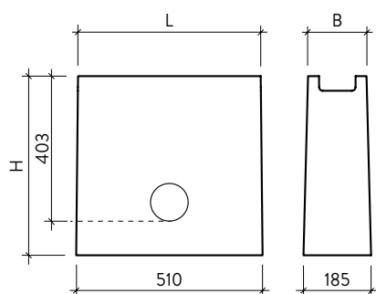
Bild 4: Liniensenkkasten Typ 1
