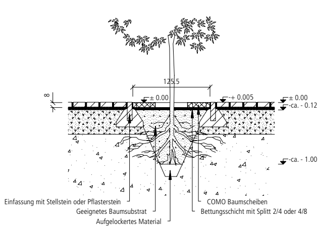
Einbauschema COMO Baumscheiben ohne Fundamentrahmen
