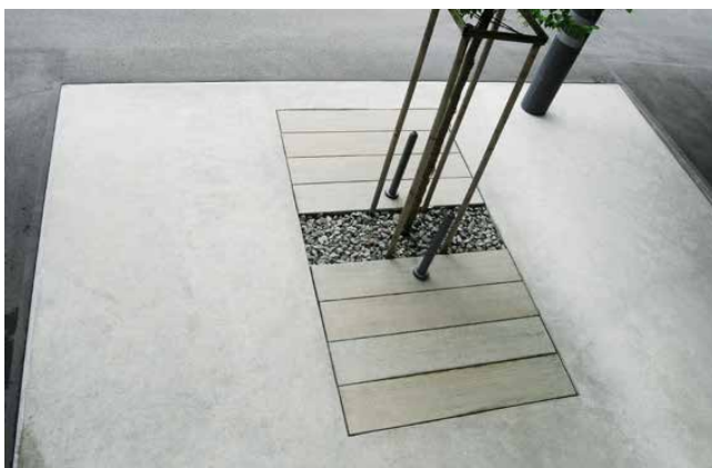
Einbau von Baumgruben mit einer Fläche von > 6 m 2
