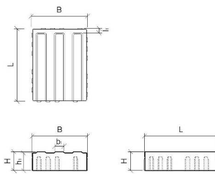
Bild 4: CARENA® Sicherheitslinienstein Typ S; H 6 cm
