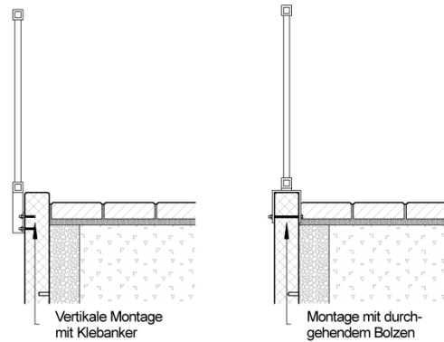
Bild 32: Mögliche Montagen von Geländer
