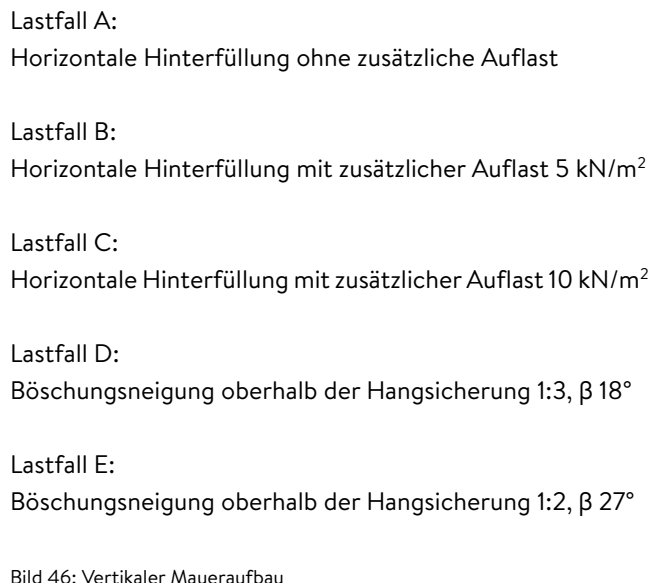
Vertikaler Maueraufbau \alpha = 90^\circ , Trockenbauweise ohne Mörtelfugen B = 25\text{ cm}
