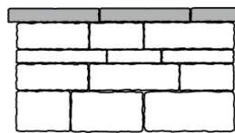
Mauertyp 12, Mauerhöhe 0,60 m
