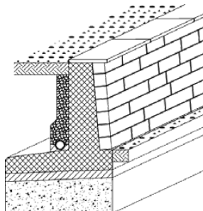
Bild 26: Stützmauer
