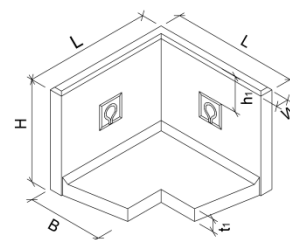
Bild 6: ROZTEC® MINI Eckelement
