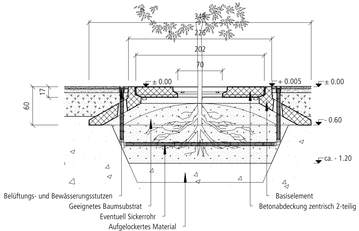
Einbauschema COPAL® CUPOLA Baumwurzelraumschutz mit Betonabdeckung zentrisch
