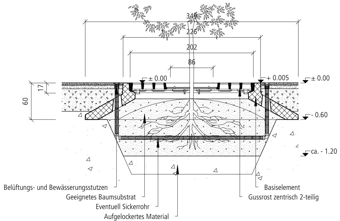
Einbauschema COPAL® CUPOLA Baumwurzelraumschutz mit Gussrost
