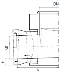
Bild 25: Anschluss mit eingebautem Muffenstück in Schachtwand
