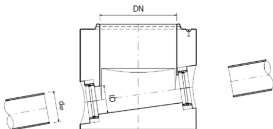
Bild 16: Anschluss mit Polyvinylchloridrohre mit Gefälle J \leq 150 ‰
