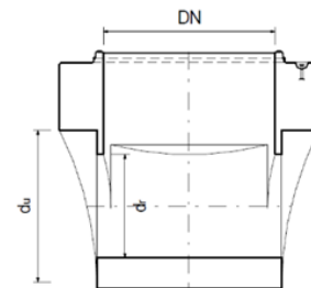
Bild 21: Aussparungen für nachträglichen Anschluss mit Bodenöffnung
