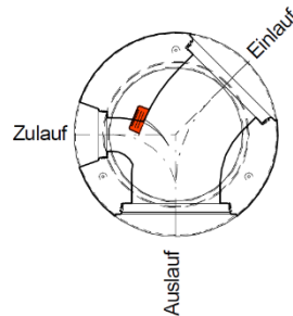
Bild 43: Definition der Platzierung der Trittnischen bei CENTUB® Massschachtunterteilen
