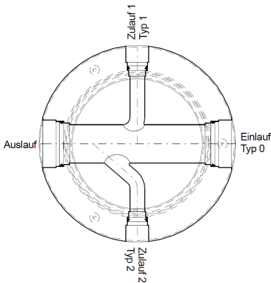
Bild 38: Bei kleinen Nennweiten ist die Anordnung eines Sohlensprunges bei CENTUB® Massschachtunterteile zu empfehlen
