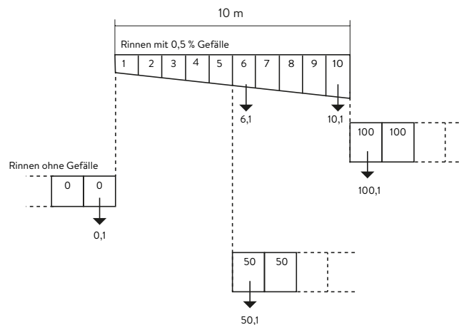
Bild 9: Rinnentypen
