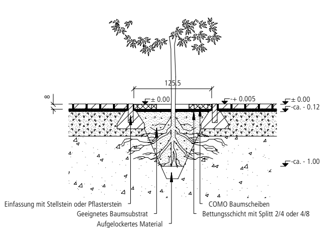
Einbauschema COMO Baumscheiben ohne Fundamentrahmen
