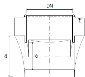
Bild 15: Anschluss mit Polyethylenrohre mit Gefälle J ≤ 500 ‰
