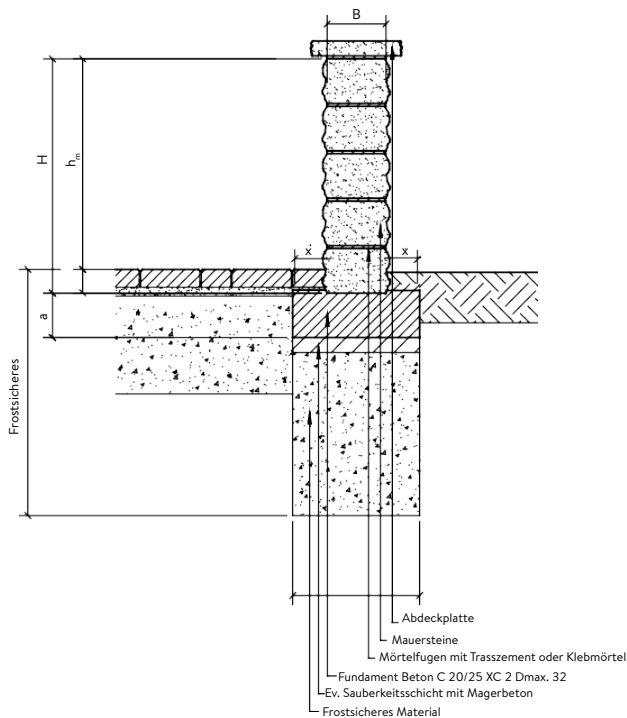
Bild 45: Freistehende Mauer, Windlast 1 \text{ kN/m}^2
