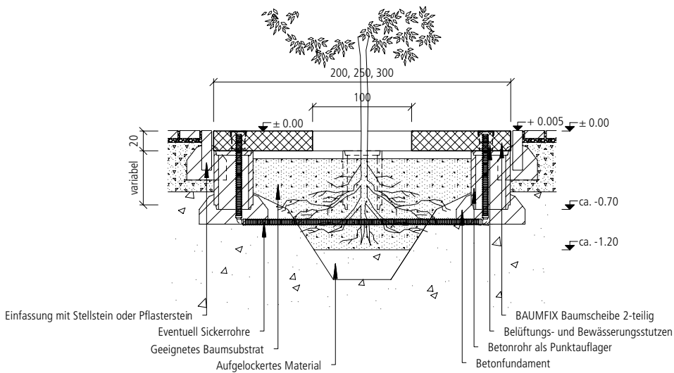
Einbauschema BAUMFIX® Baumscheiben auf Punktaufleger (z. B. Betonrohre DN 300)
