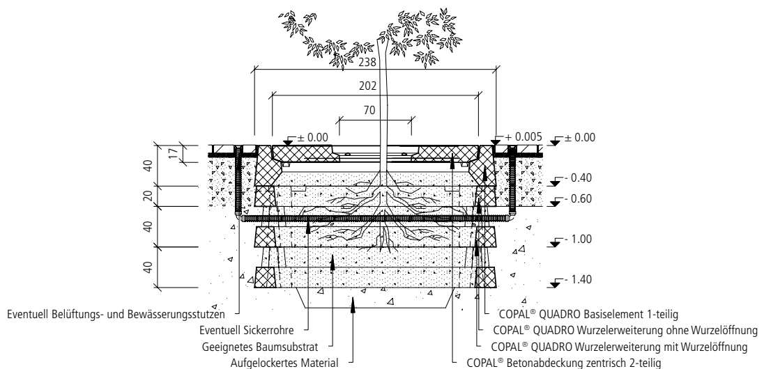
Einbauschema COPAL® QUADRO Baumwurzelraumschutz mit Betonabdeckung exzentrisch und Wurzelraumerweiterung mit Wurzelöffnungen
