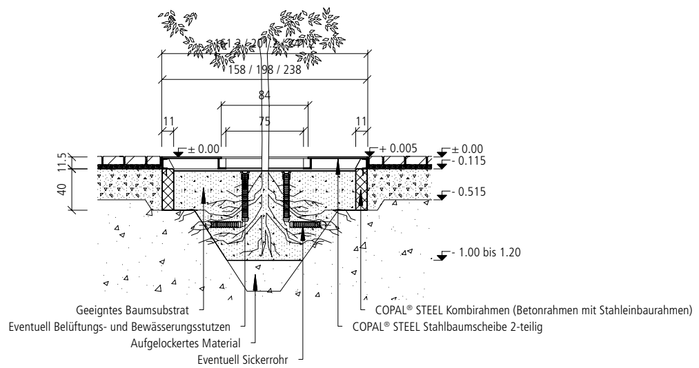
Einbauschema COPAL® STEEL Stahlbaumscheibe mit Kombirahmen
