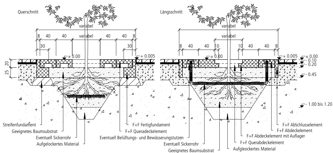
Einbauschema F+F Baumwurzelraumschutz mit Fertigteilfundamenten und Abschlusselementen
