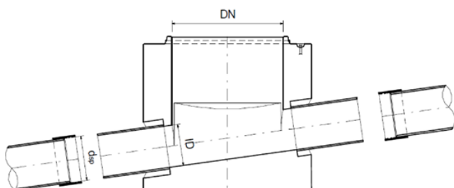
Bild 19: Anschluss mit glasfaserverstärkten ungesättigten Polyesterrohren mit Gefälle mit Gefälle J \leq 500 \text{ ‰}
