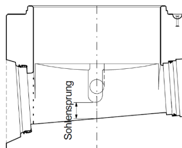
Bild 39: Bei kleinen Nennweiten ist die Anordnung eines Sohlensprunes bei CENTUB® Massschachtunterteil zu empfehlen
