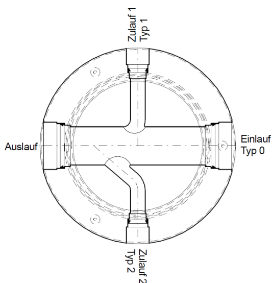
Bild 38: Bei kleinen Nennweiten ist die Anordnung eines Sohlensprunes bei CENTUB® Massschachtunterteil zu empfehlen
