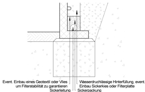
Bild 22: Mögliche Lage einer Sickerleitung
