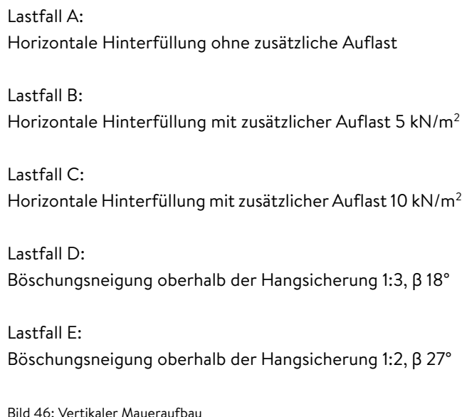
Vertikaler Maueraufbau \alpha = 90^\circ , Trockenbauweise ohne Mörtelfugen B = 25 cm
