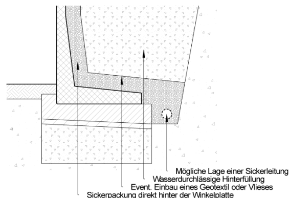
Bild 28: Mögliche Lage einer Sickerleitung
