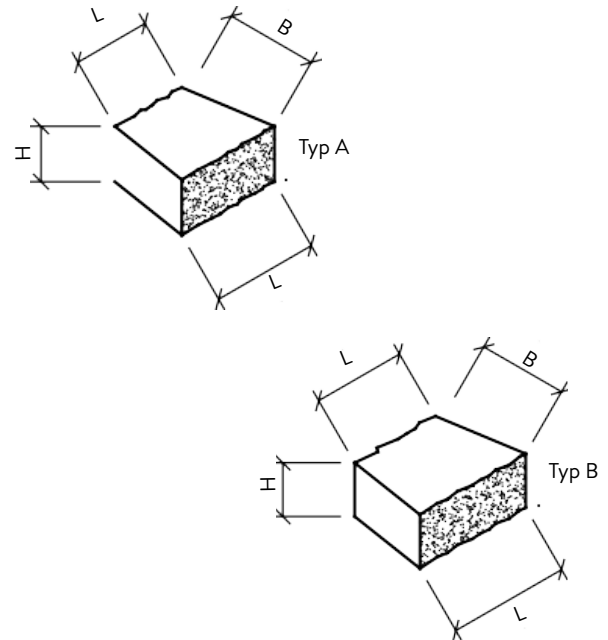
Bild 16: Technische Zeichnung SANTURO® Spaltkeilmauerstein 2seitig gespalten
