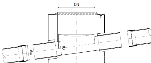
Bild 13: Anschluss mit Polypropylenrohren mit Gefälle J ≤ 500 ‰
