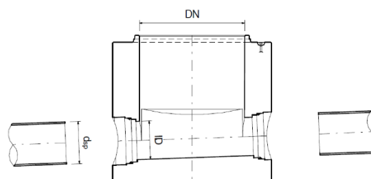
Bild 12: Anschluss mit Polypropylenrohren mit Gefälle J ≤ 150 ‰
