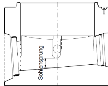
Bild 39: Bei kleinen Nennweiten ist die Anordnung eines Sohlensprungs bei CENTUB® Massschachtunterteilen zu empfehlen
