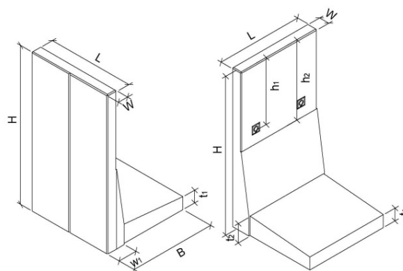
Bild 6: EXACTA® Winkelplatte Typ 2
