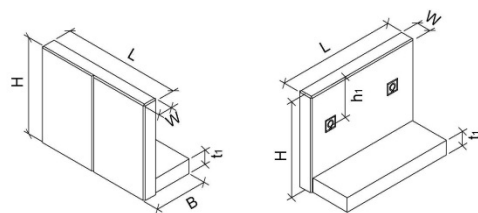
Bild 4: EXACTA® Winkelplatte Typ 1
