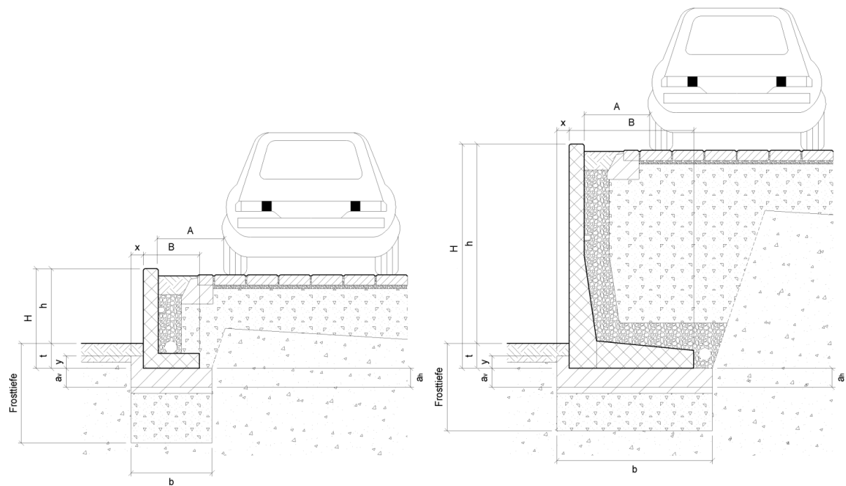
Bild 39: Fundamentabmessungen für Lastfall B2, A = 20 cm
