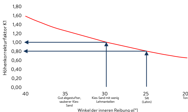
Diagramm 1: Höhenkorrekturfaktor K1
