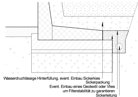
Bild 21: Mögliche Lage einer Sickerleitung
