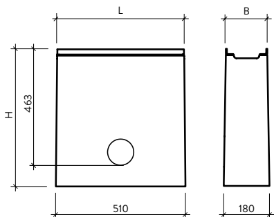
Bild 4: Liniensinkkasten Typ 1
