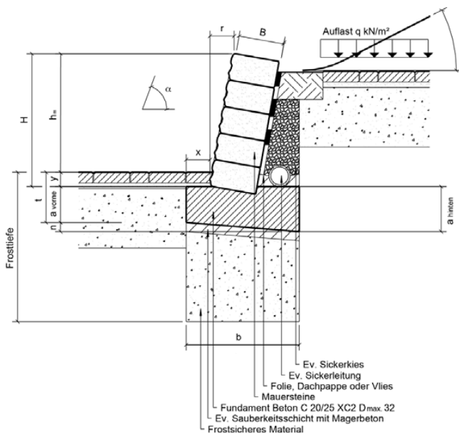
Bild 47: Geneigter Maueraufbau
