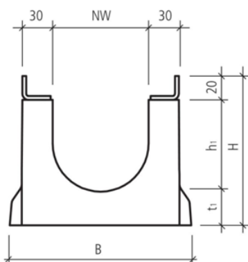
Bild 2: Geometrie BIRCOLight®
