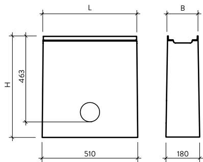
Bild 4: Liniensinkkasten Typ 1
