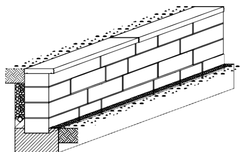
Bild 26: Stützmauer
