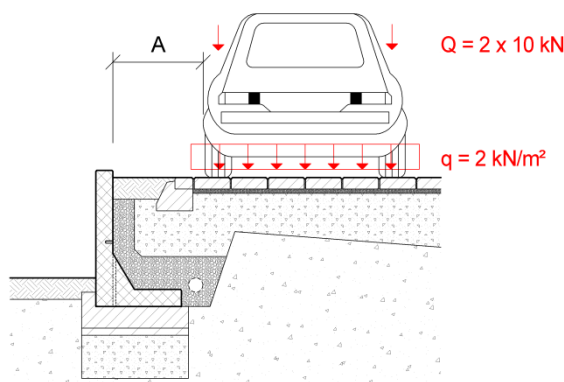
Bild 9: Lastfall B2
