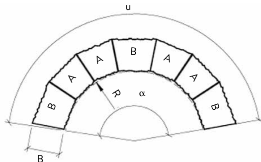
Bild 31: Optimale Muffenbildung
