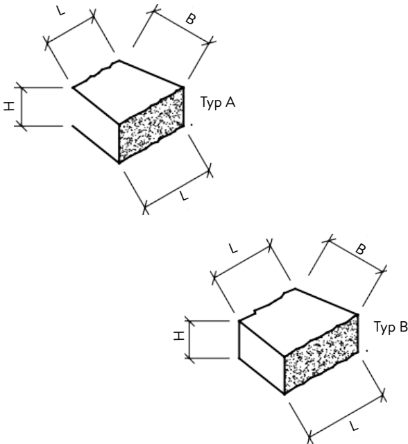
Bild 16: Technische Zeichnung SANTURO® Spaltkeilmauerstein 2seitig gespalten
