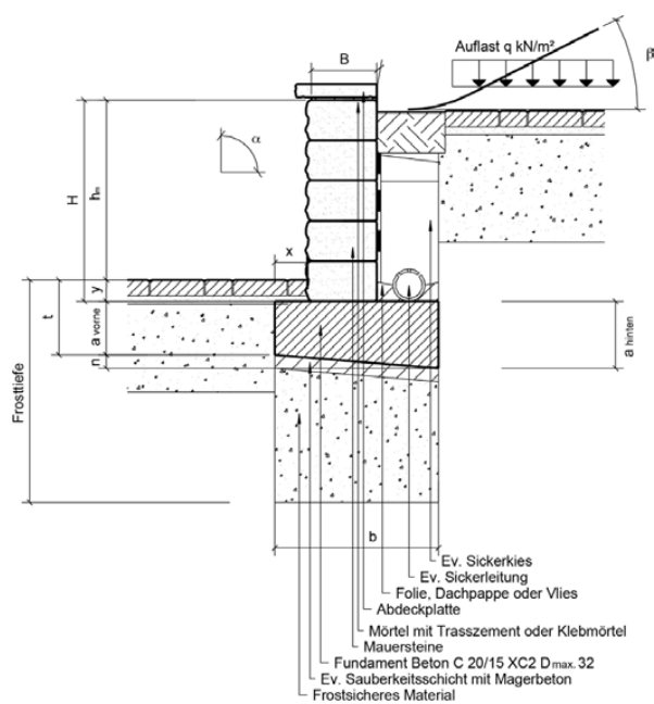
Bild 40: Aufbauquerschnitt
