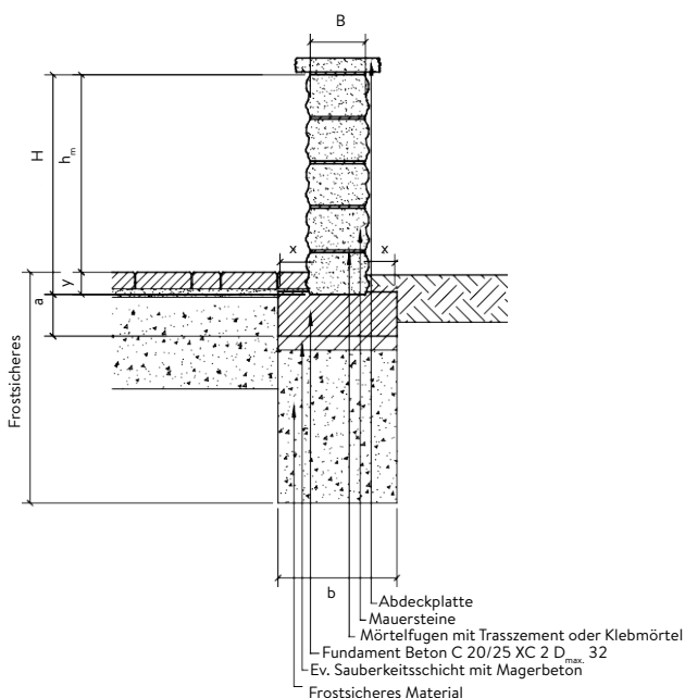
Bild 45: Freistehende Mauer, Windlast 1 \text{ kN/m}^2
