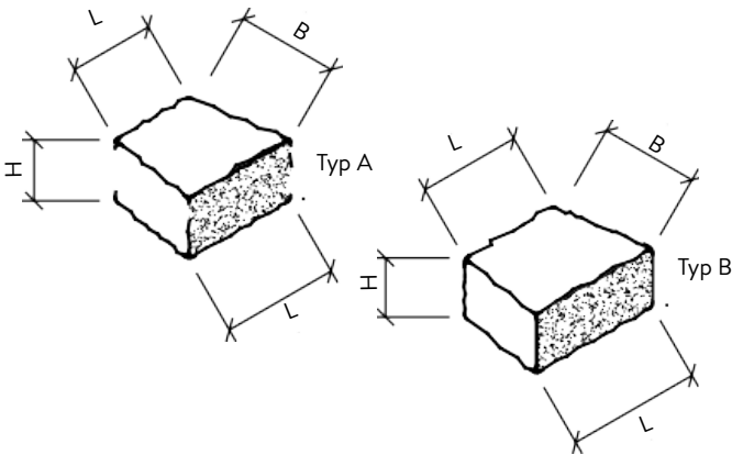
Bild 18: Technische Zeichnung SANTURO® Weinbergkeilmauerstein 2seitig gespalten, Kanten gebrochen
