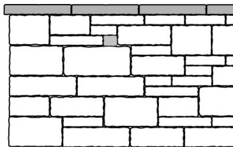
Mauertyp 20, Mauerhöhe 0,98 m
