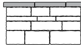
Mauertyp 12, Mauerhöhe 0,60 m
