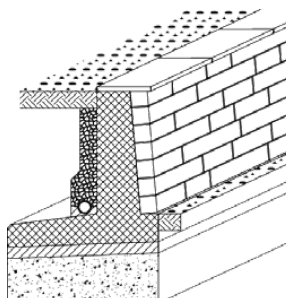
Bild 26: Stützmauer
