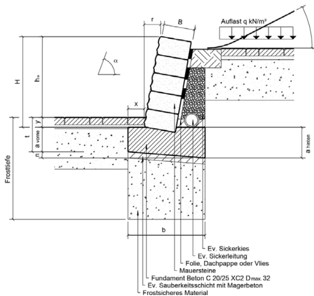
Bild 47: Geneigter Maueraufbau
