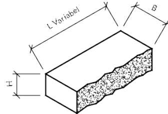
Bild 8: Techn. Zeichnung SANTURO® Spaltmauerstein 1seitig gespalten
