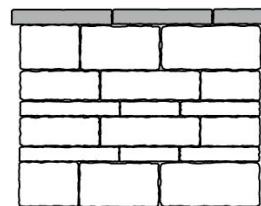
Mauertyp 15, Mauerhöhe 0,90 m
