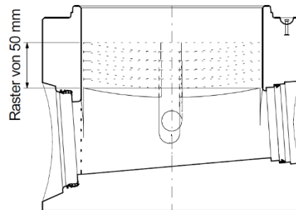
Bild 40: Mögliche Erhöhung der Auftritte bei CENTUB® Massschachtunterteilen
