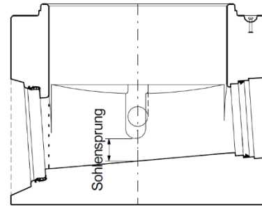
Bild 39: Bei kleinen Nennweiten ist die Anordnung eines Sohlensprunges bei CENTUB® Massschachtunterteil zu empfehlen
