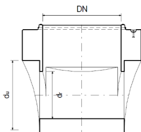
Bild 15: Anschluss mit Polyethylenrohre mit Gefälle J \leq 500 ‰
