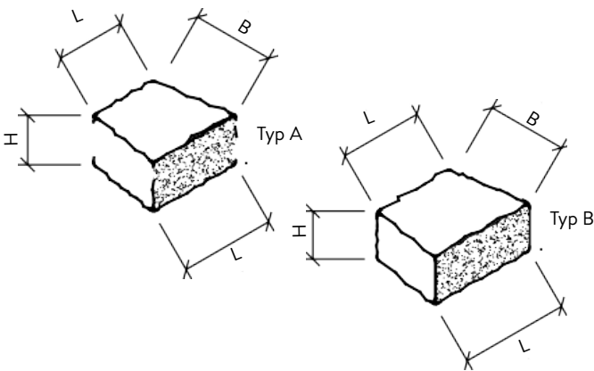
Bild 18: Technische Zeichnung SANTURO® Weinbergkeilmauerstein 2seitig gespalten, Kanten gebrochen
