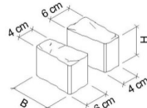
FRIEDA® Pflastersteine 4/6 × 9.8 × 7 cm (Keilsteine)
