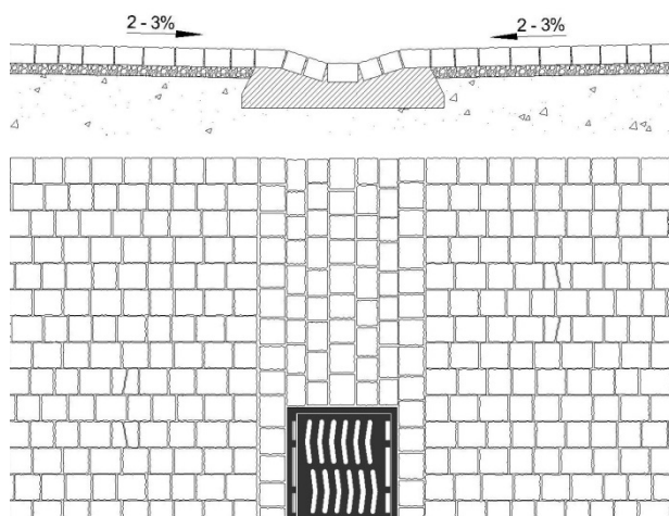
Mögliche Rinnenausbildung mit FRIEDA® Pflastersteinen
