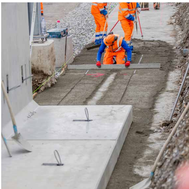
Erstellung des Streifenfundamentes
