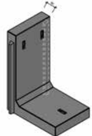
GRANDE Winkelplatte W = 25 cm
