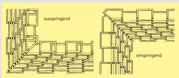
Eckenabwicklung
