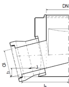
Bild 28: Anschluss mit eingebautem Muffenstück in Schachtwand, Muffenstück bis unter die Sohle
