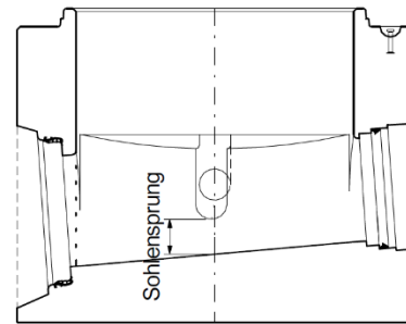
Bild 39: Bei kleinen Nennweiten ist die Anordnung eines Sohlensprungs bei CENTUB® Massschachtunterteil zu empfehlen
