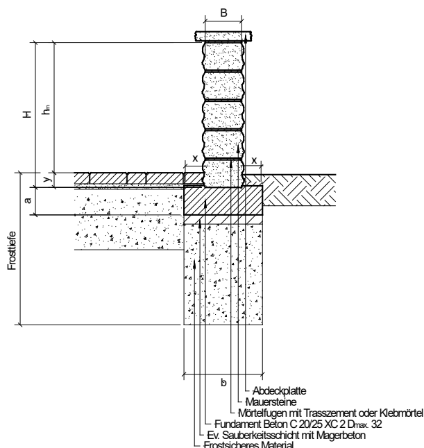
Freistehende Mauer, Windlast 1 kN/m 2 , Trockenbauweise ohne Mörtelfugen B = 25 cm
