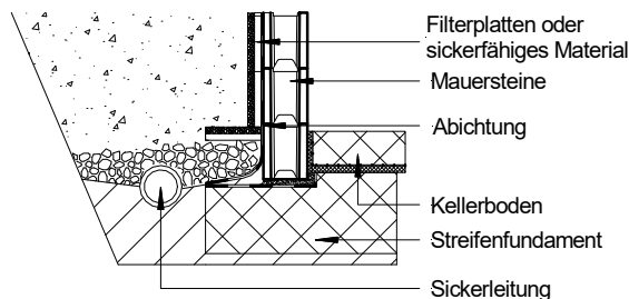
Bild 18 Entwässerung
