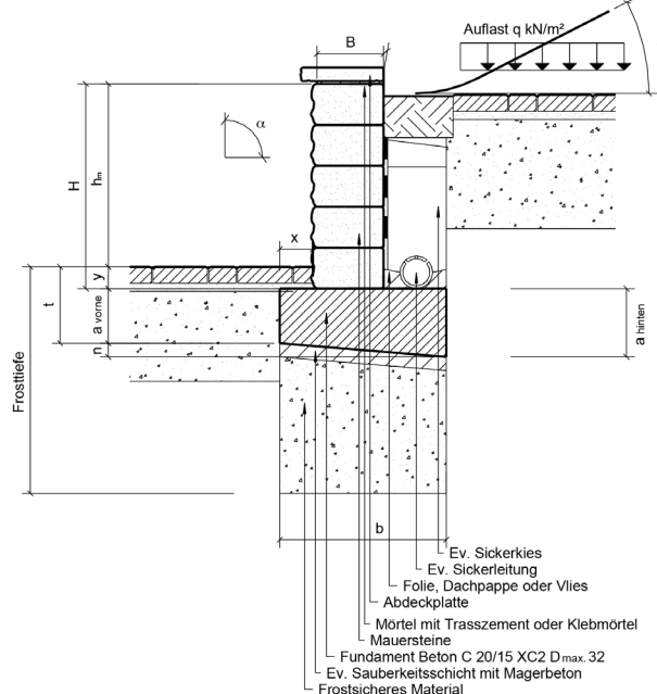
Bild46: Vertikaler Maueraufbau
