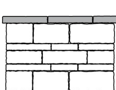
Mauertyp 14, Mauerhöhe 0.75 m
