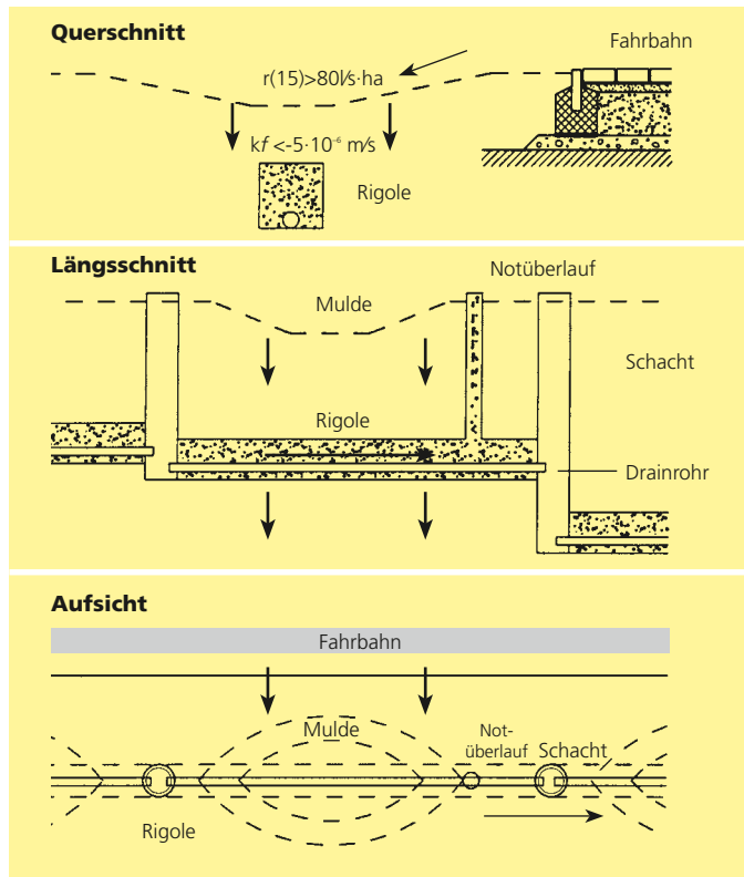
Prinzipskizze Mulden-Rigolen-System
