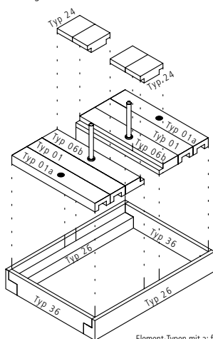
Verlegeart C
