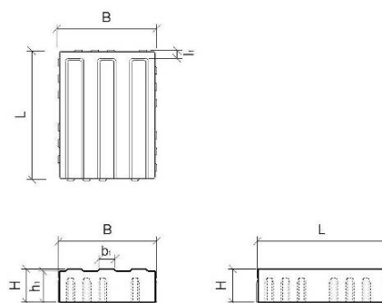
Bild 4: CARENA® Sicherheitslinienstein Typ S; H 6 cm
