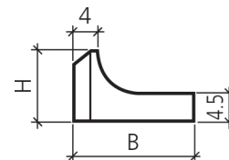
Bild 7: Abschlussbalken unten
