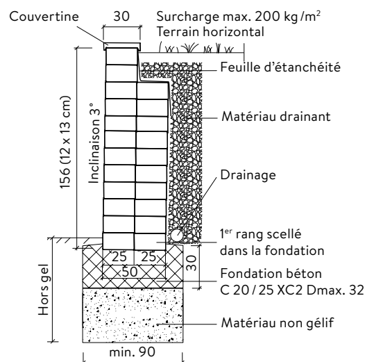
Exemple de réalisation d'un mur sans géogrid, épaisseur = 50 cm
