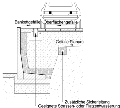
Bild 23: Zusätzliche Entwässerung
