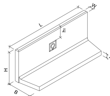
Bild 4: ROZTEC® MINI Winkelplatte
