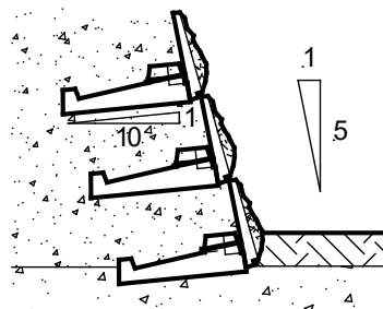
Bild 34: Aufbau 1:5
