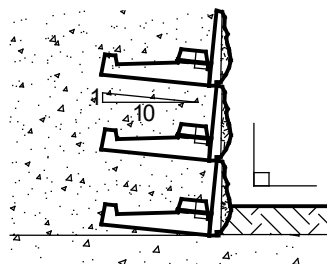
Bild 32: Vertikaler Aufbau
