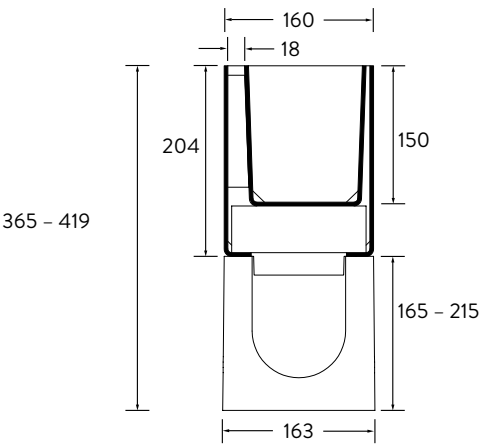
Illustration 11 : type asymétrique
